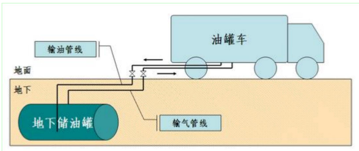
图 2-2 卸油油气回收系统示意图
