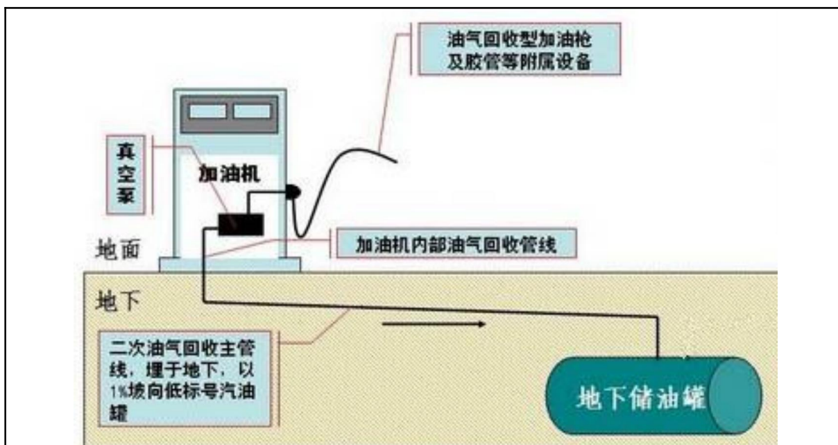
2-3 加油油气回收系统示意图
