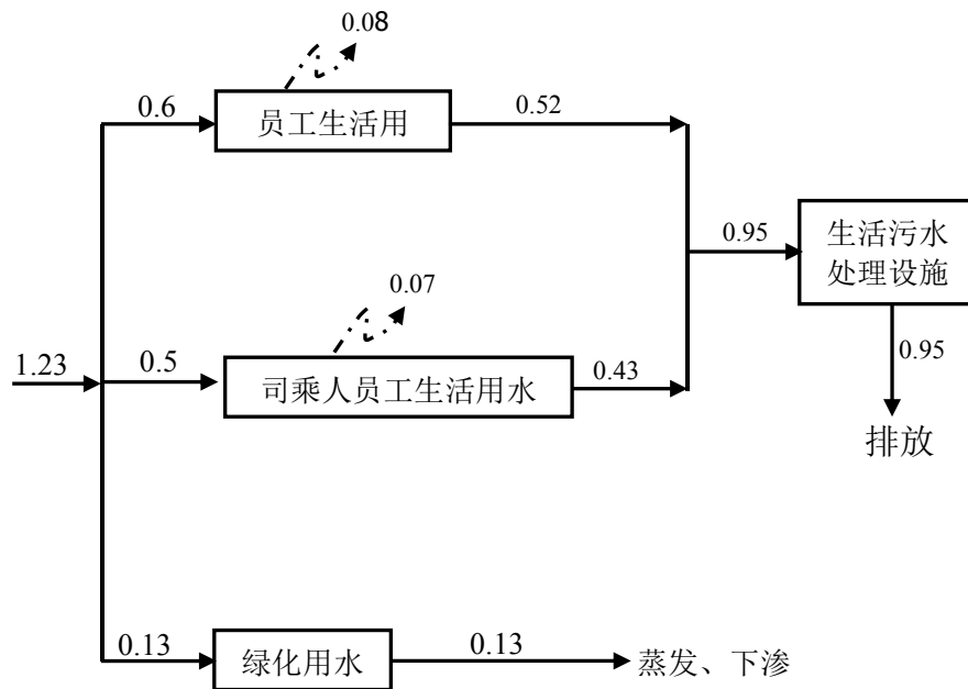
图 2-1 本项目水平衡图 单位: t/d
