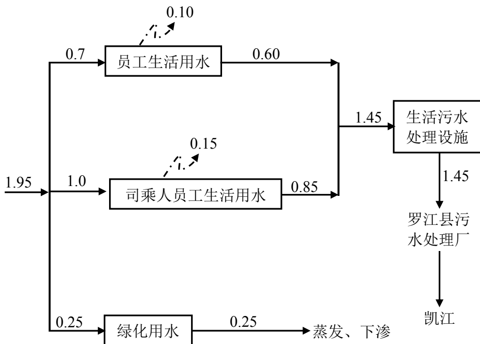
图 2-1 本项目水平衡图 (m 3 /d)
